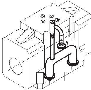
Condotti drenaggio
