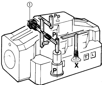
Condotti pilotaggio
