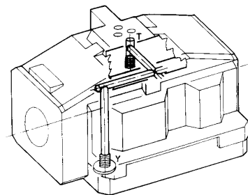
Condotti drenaggio
