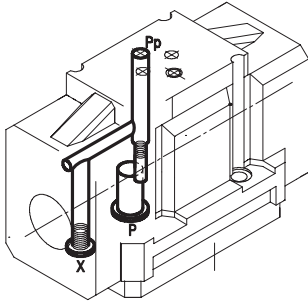
Condotti pilotaggio
