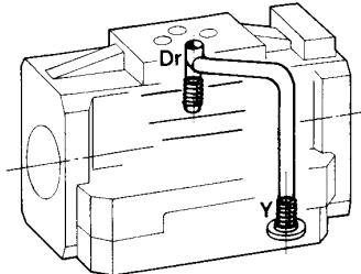
Condotti drenaggio
